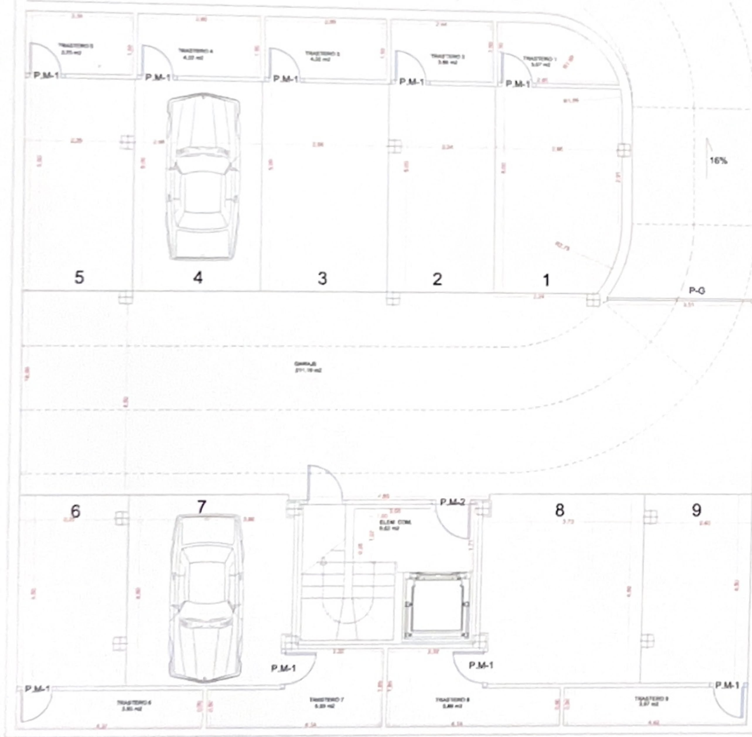
PLANTA SÓTANO
